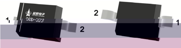
PIN1:Cathode PIN2:Anode
